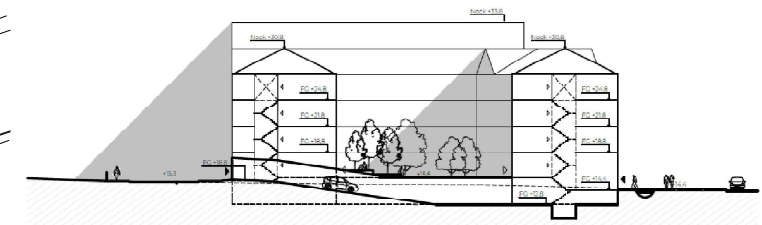
Sektion B-B
